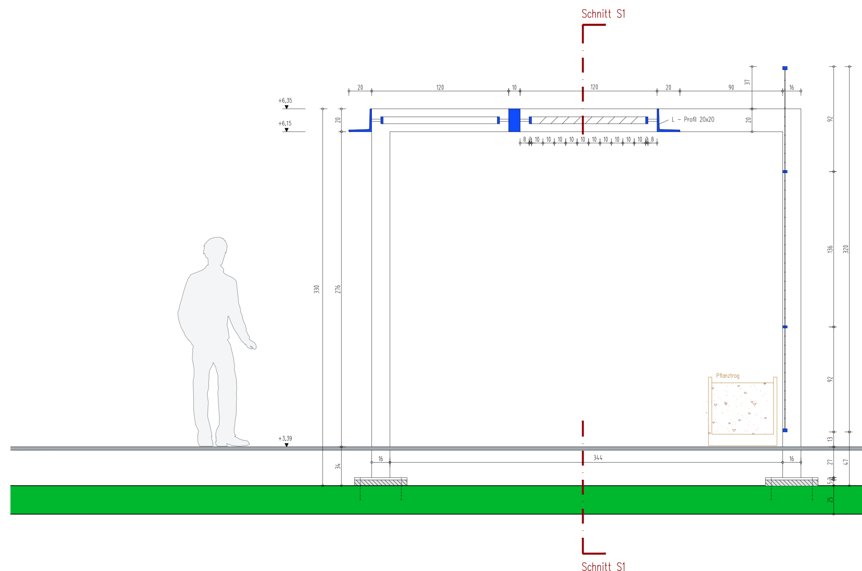
SCHNITT S2 PERGOLA OG - M 1:20
